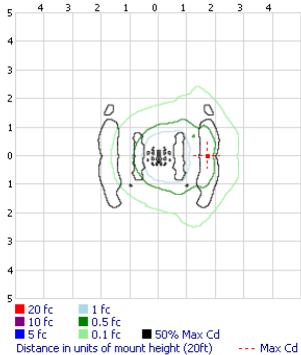
Isofootcandle Plot
