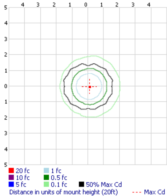
Isofootcandle Plot
