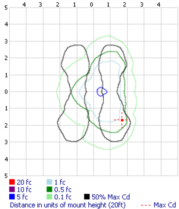
Isofootcandle Plot
